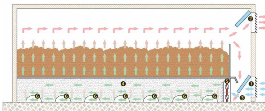
Рисунок 1– Схема вентилирования овощехранилища
