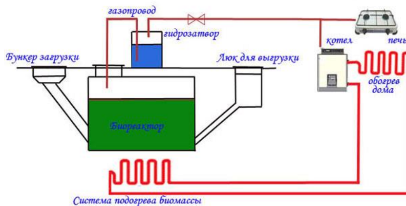
Рис.2 - Биогазовая установка в подогревом биомассы [1]
