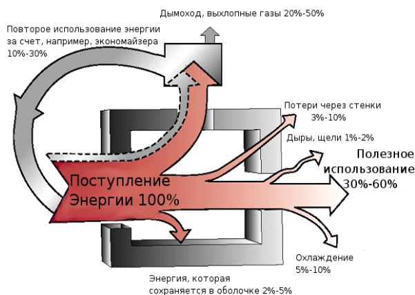
Рисунок 1. Диаграмма энергетического баланса предприятия.
