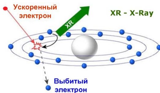
Рисунок 1 – Сущность рентгенофлуоресцентного анализа
