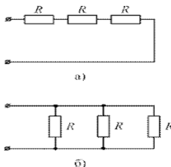
Рисунок 1 – Соединение резисторов
