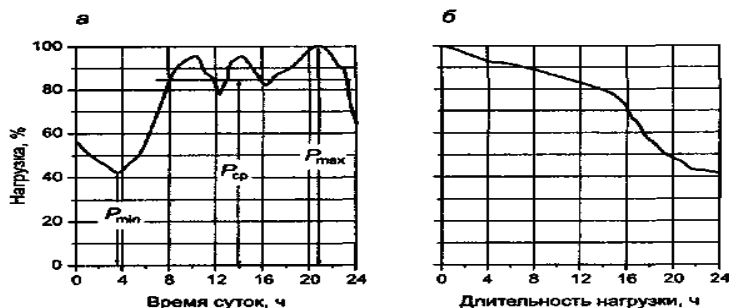
Рисунок 1 -Изменение нагрузки
